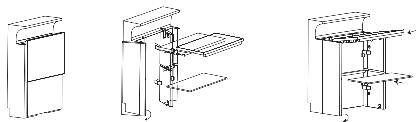
Modulo chiuso Closed element Aprire le due ante e inserire il piano Open the two sides and place the top Inserire la mensola Place the shelf
